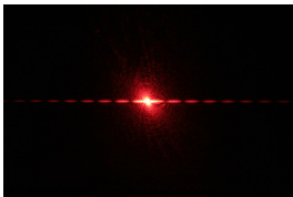
Diffraction de la lumière par une fente
